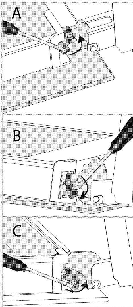
Sarnyro užraktas - uždaryta padėtis
