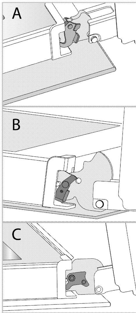
Sarnyro užraktas - atidarymo padėtis 3. Perkelti orkaitės dureles į pusiau atidarytą padėtį.
