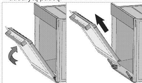
Sarnyro užraktas - atidarymo padėtis 3. Perkelti orkaitės dureles į pusiau atidarytą padėtį.
